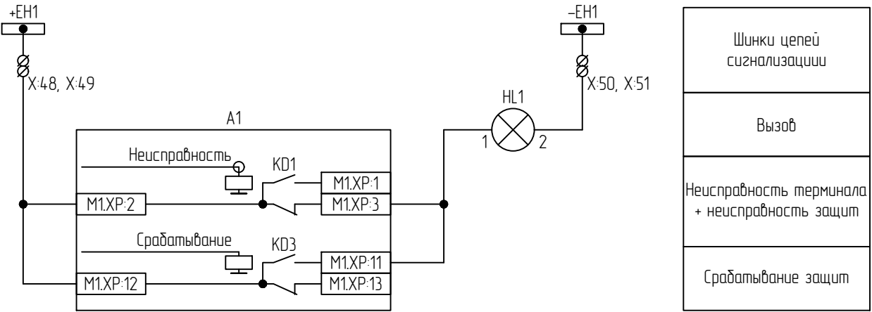
Цепи сигнализации
