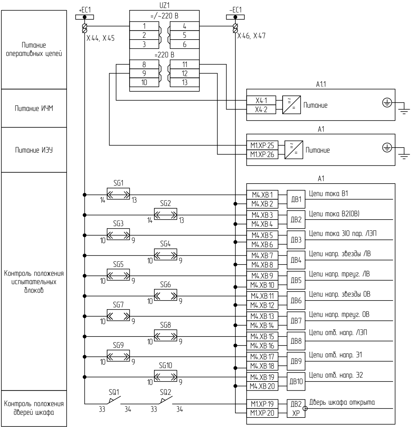
Цепи оперативного тока
