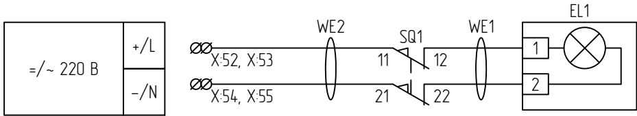
Цепи освещения
